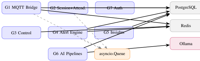
Fig. 6. Backend internal module diagram.
