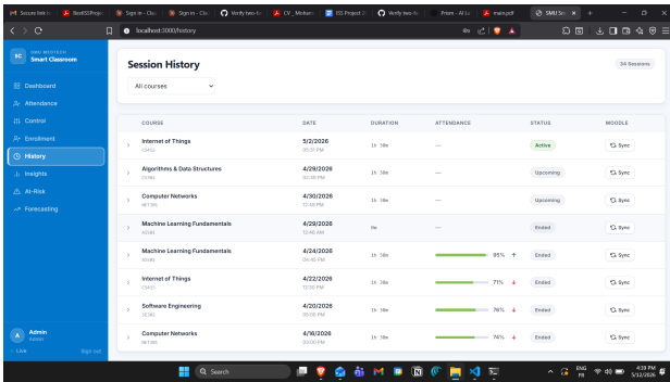
Fig. 15. History page.
