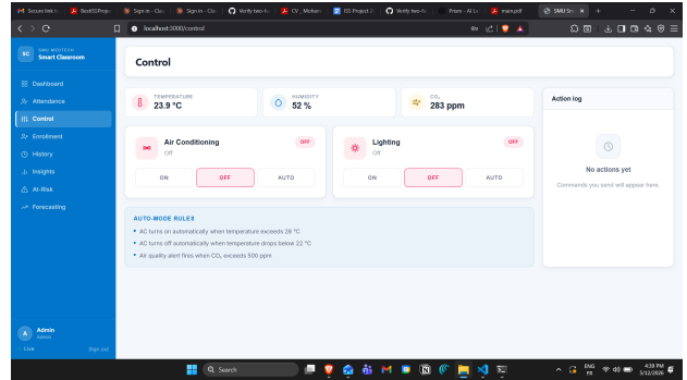
Fig. 11. Control page.
