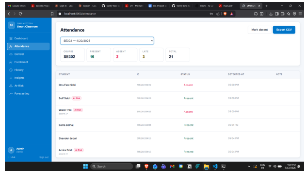
Fig. 10. Attendance page.
