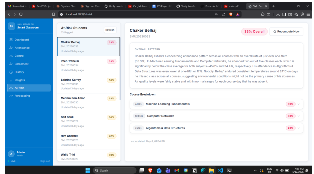
Fig. 12. At-Risk page.
